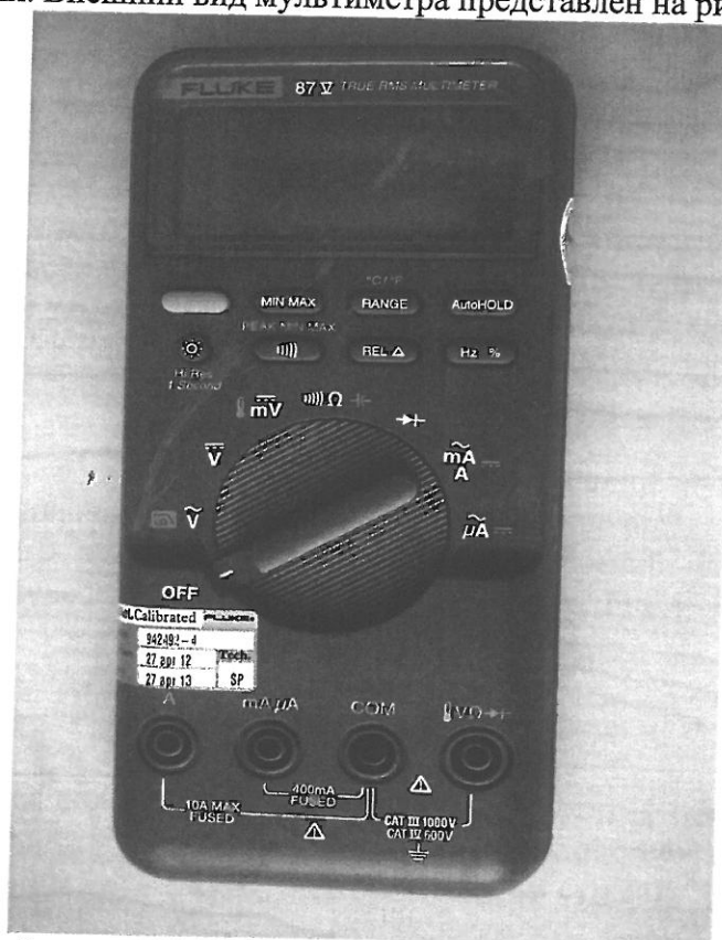
Рисунок 1 - Внешний вид мультиметра Fluke 87V.
