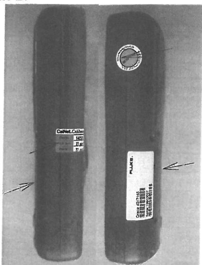
Рисунок 2 - Места пломбирования от несанкционированного доступа, показаны стрелками на боковых сторонах, на нижней поверхности мультиметра стрелкой показано место нанесения знака утверждения типа.
